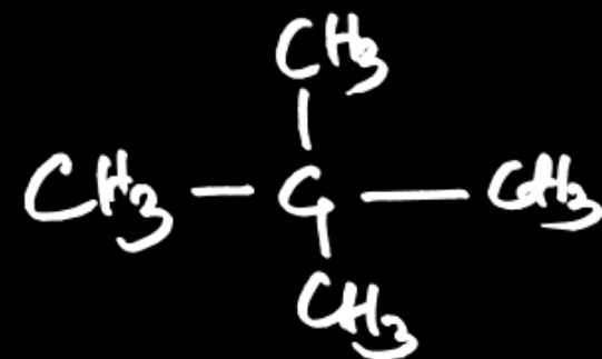
neo-pentane त्रि-मेथेन
