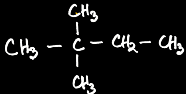
neo-hexane त्रि-मेथेन
